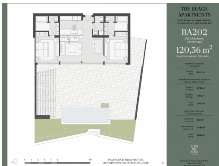
Grundriss Wohnung
