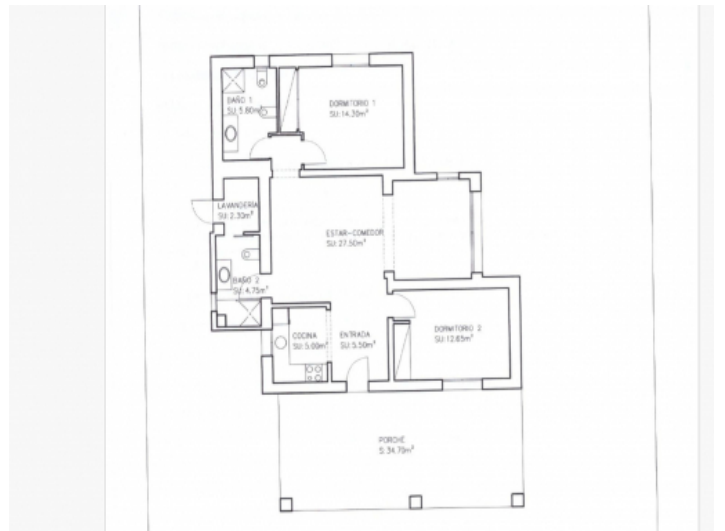
Grundriss Gästehaus
