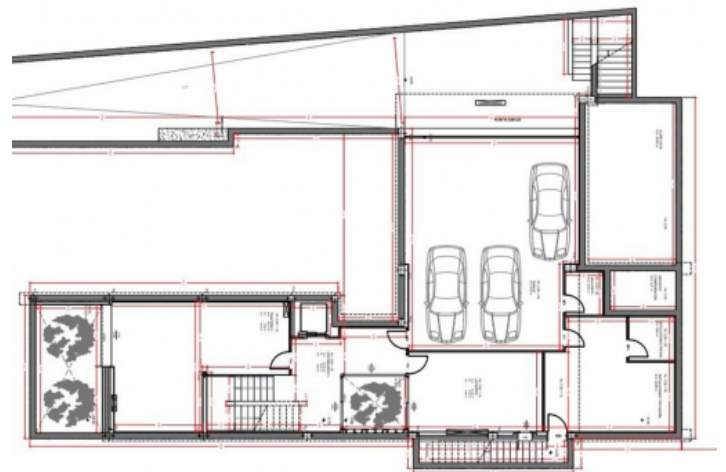
Grundriss Keller
