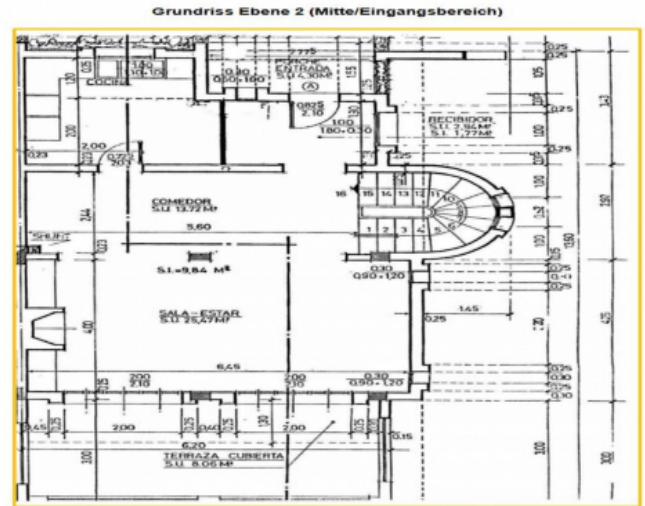
Grundriss OG
