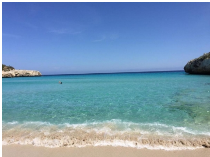
Cala Murada
