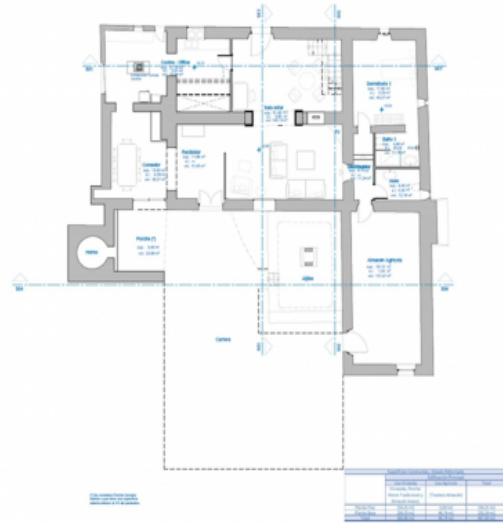
Grundriss Erdgeschoss
