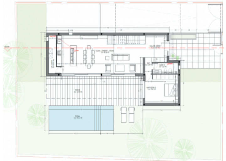
Pläne Erdgeschoss
