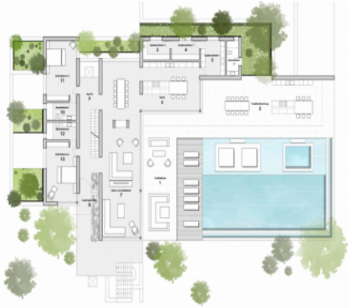
Grundriss Erdgeschoss
