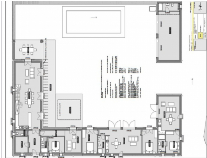
Grundriss
