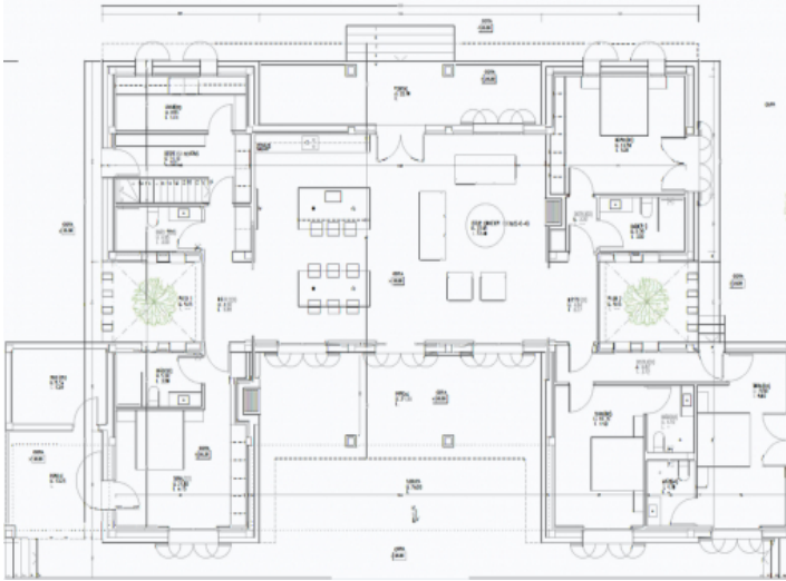
Grundriss vom Hausprojekt
