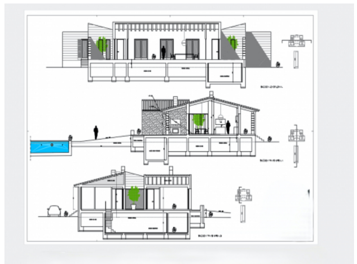
Schnittzeichnung
